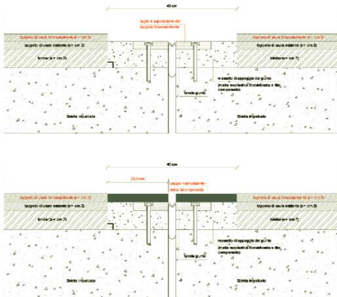
FIG. 5 Asportazione del conglomerato in prossimità dei giunti e successiva posa di cappa insonorizzante
